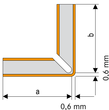
Abb. Außenecke 90°
