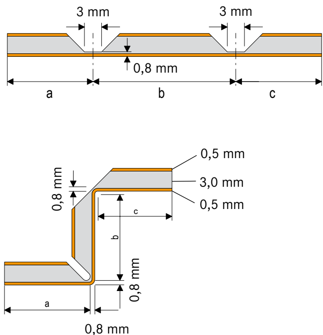
Abb. Innen- und Außenecke 90°
