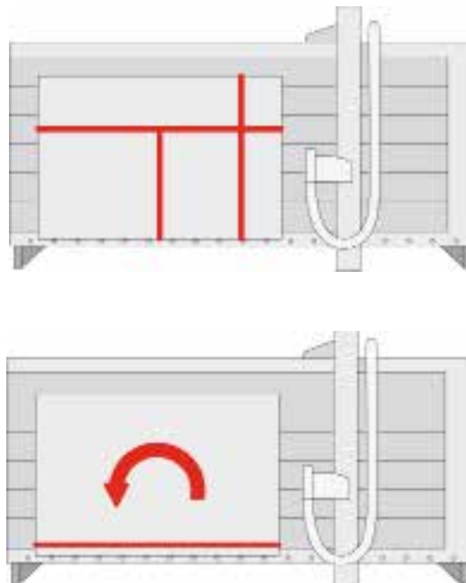
Abb. Plattensäge - auf der Plattenrückseite arbeiten
