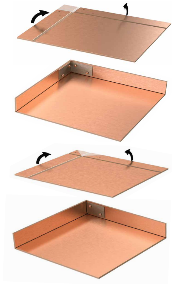
Beispiele für die Anordnung des Niet in Abhängigkeit der Eckausschnitte bei umlaufend aufgekanteten Formaten
